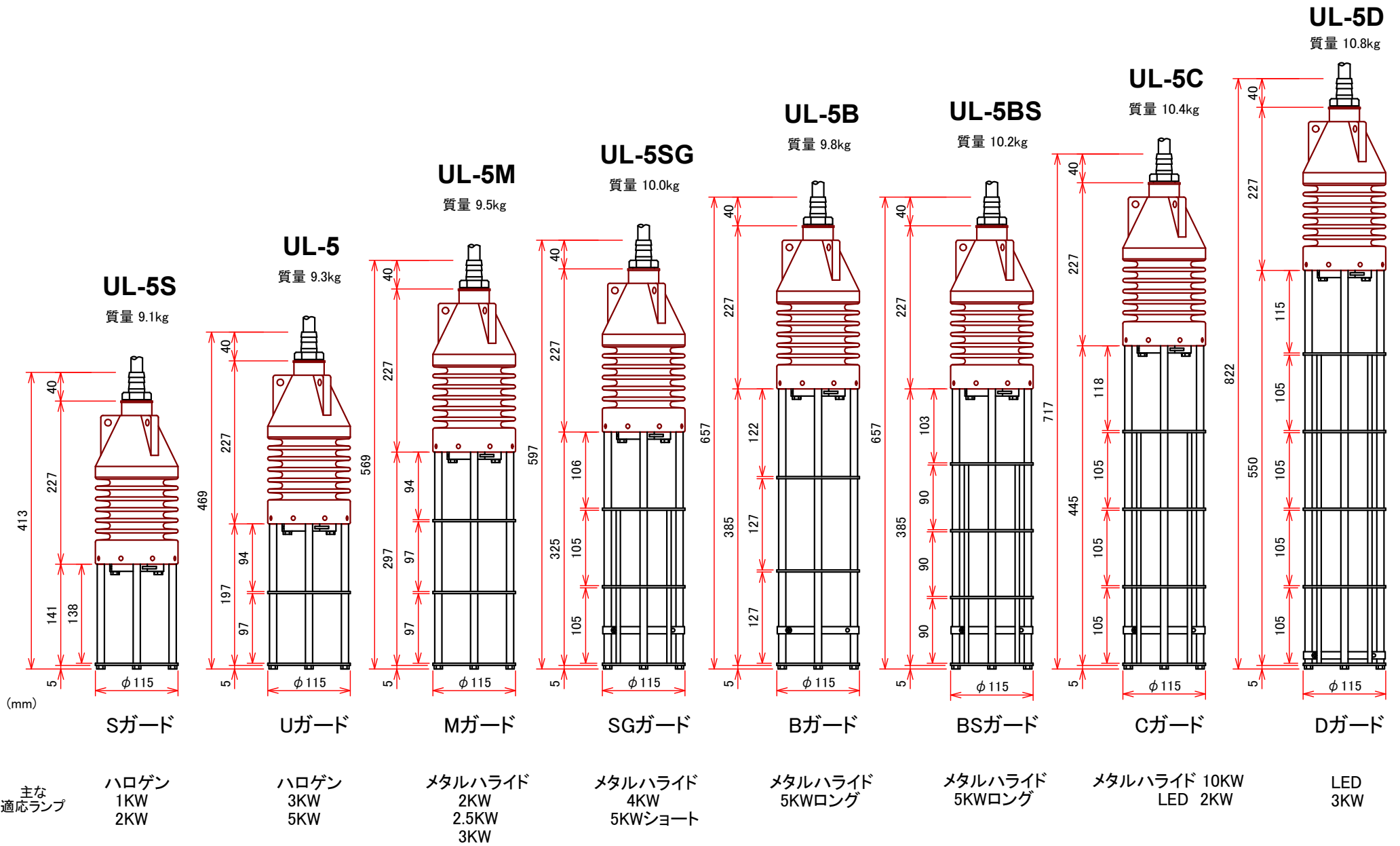
UL灯具5型(UL-5) 外形寸法一覧
