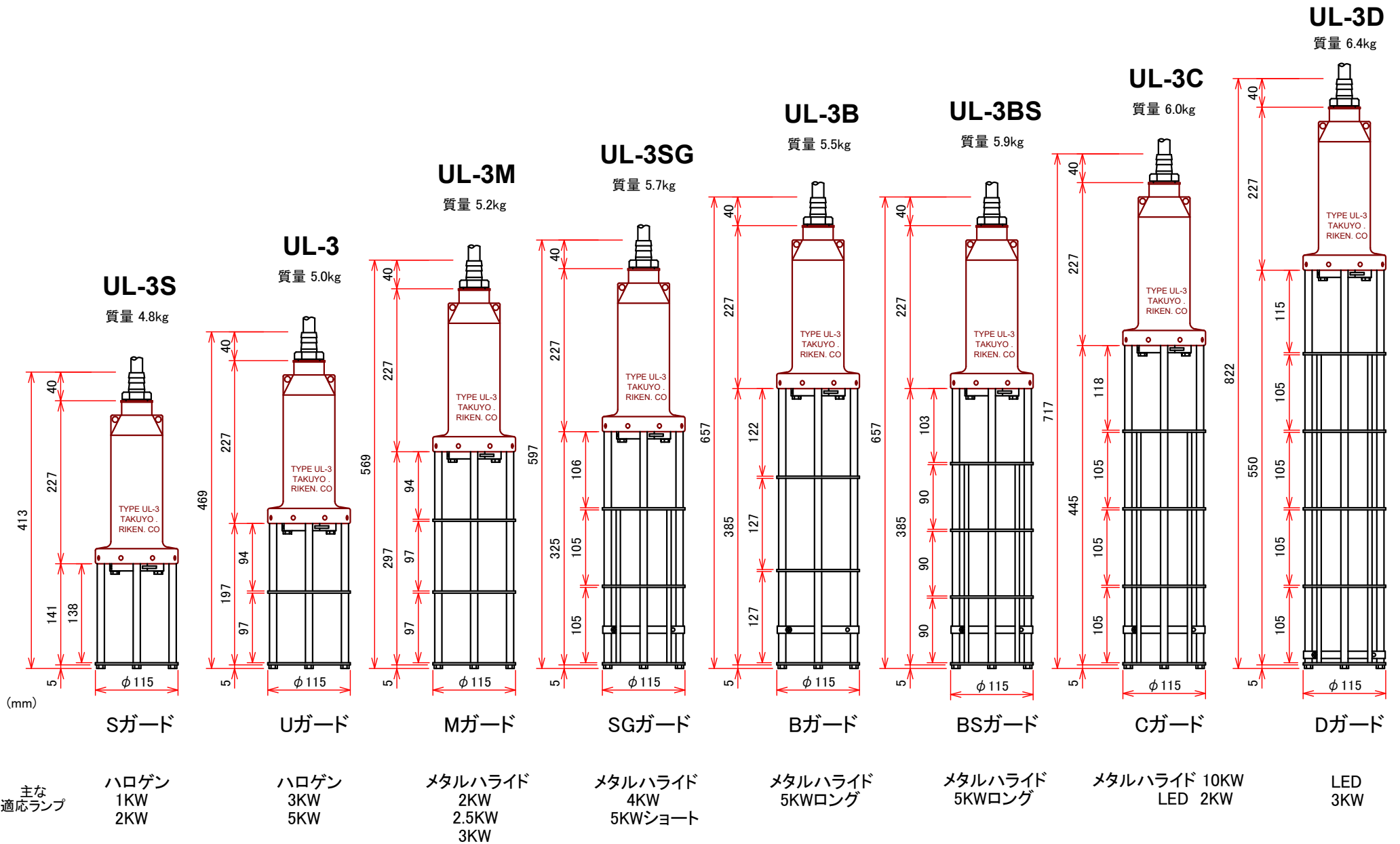
UL灯具3型(UL-3) 外形寸法一覧
