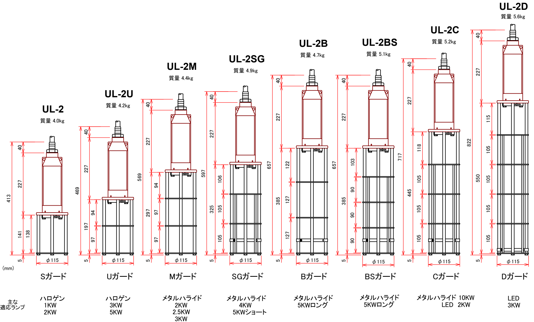
UL灯具2型(UL-2) 外形寸法一覧
