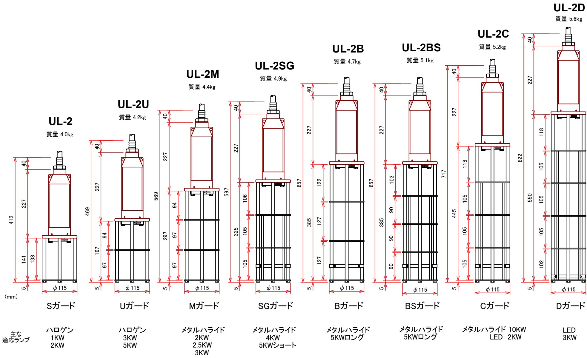
UL灯具2型(UL-2) 外形寸法一覧
