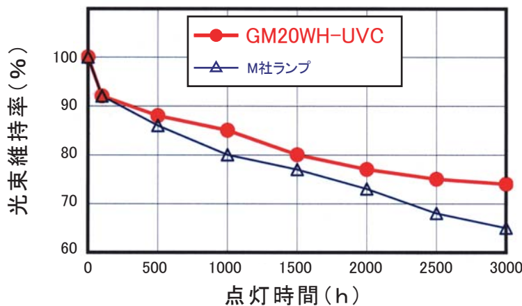
ランプ電力2000Wで寿命試験したときの光束維持率
