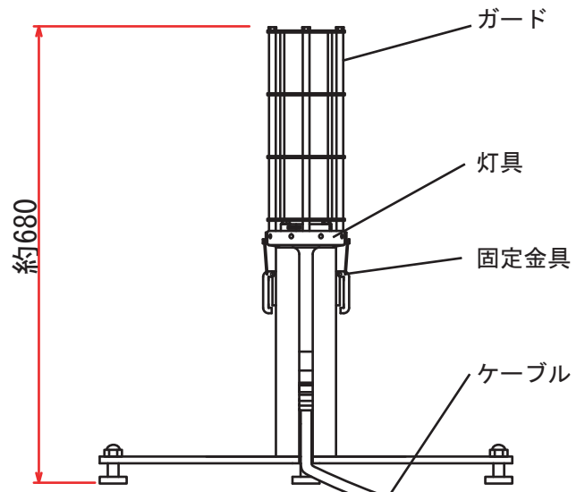
水中灯固定スタンド外形図
